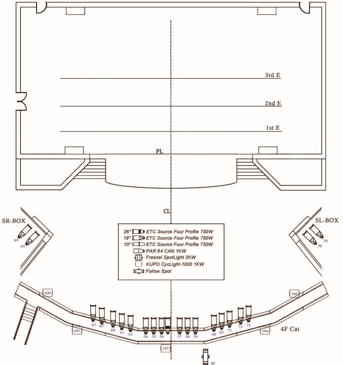
燈具配置圖
