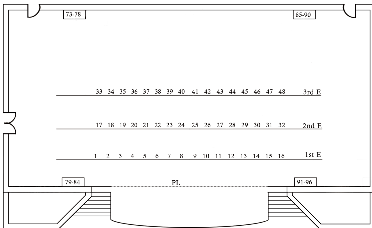
舞台區燈光迴路配置
