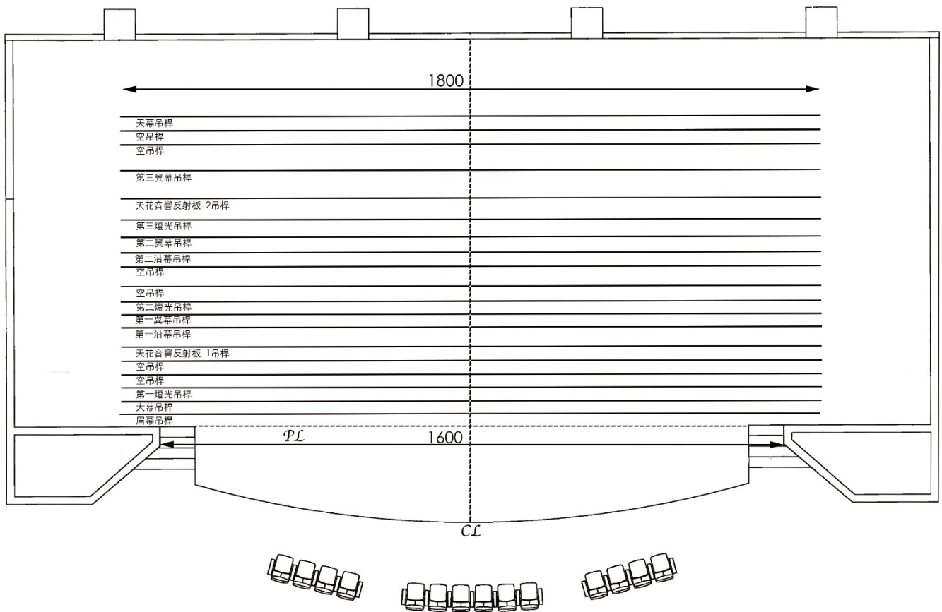
懸吊平面圖
