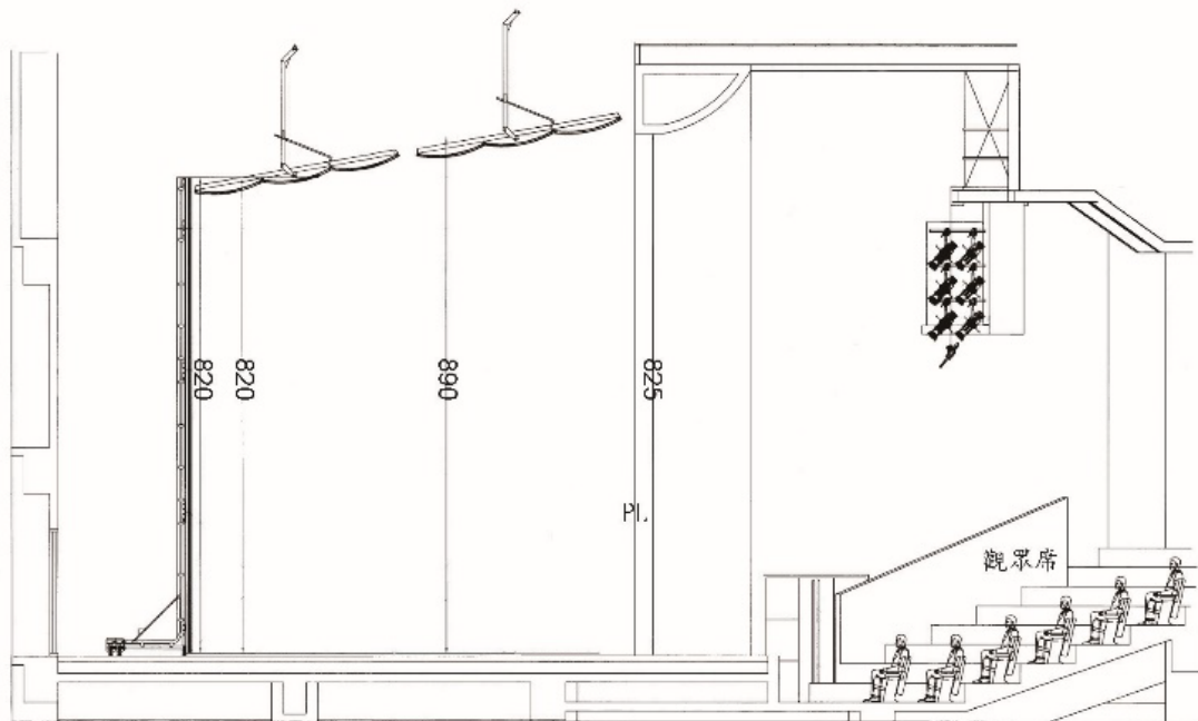
反射板剖面圖
