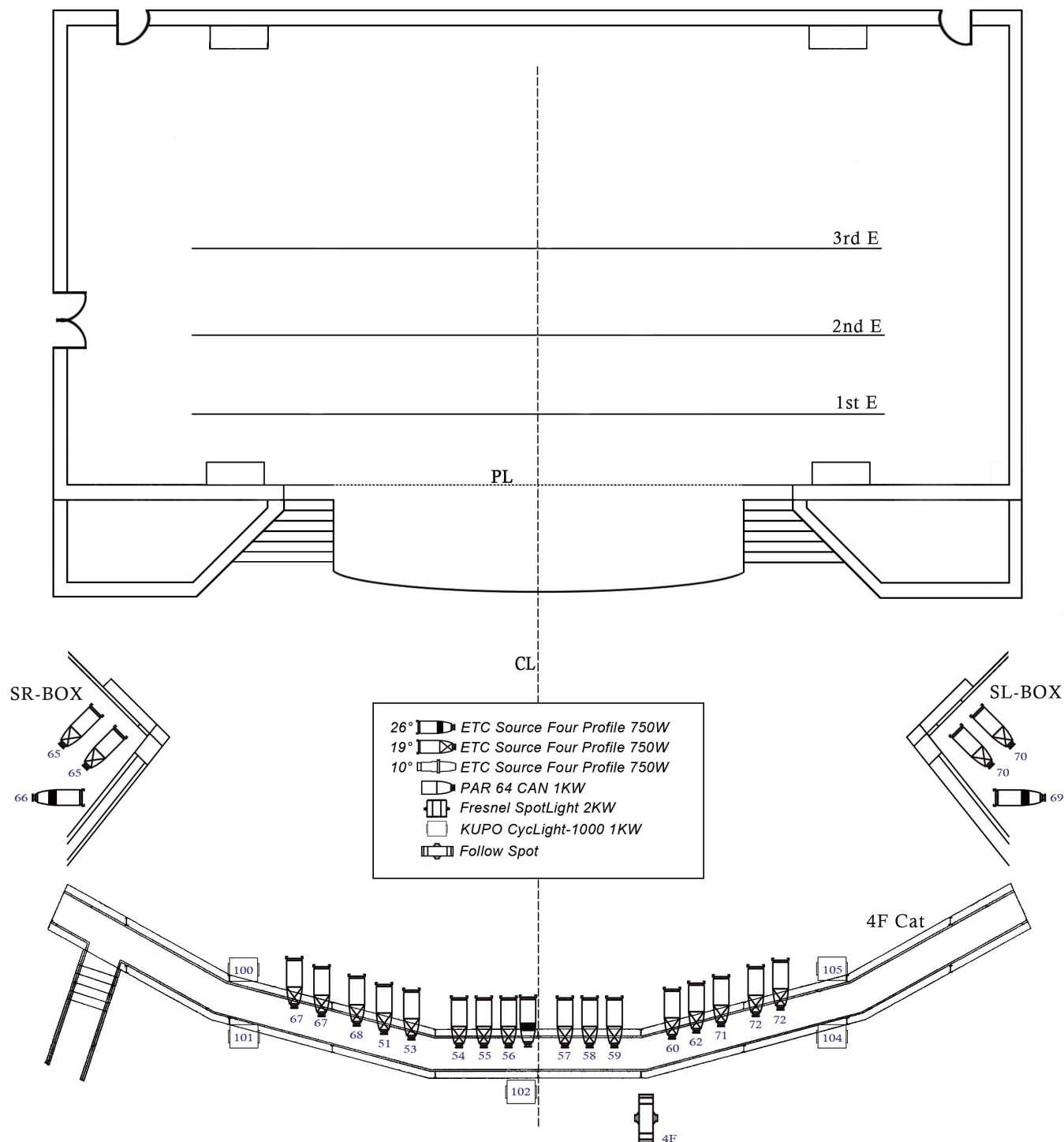
燈具配置圖
