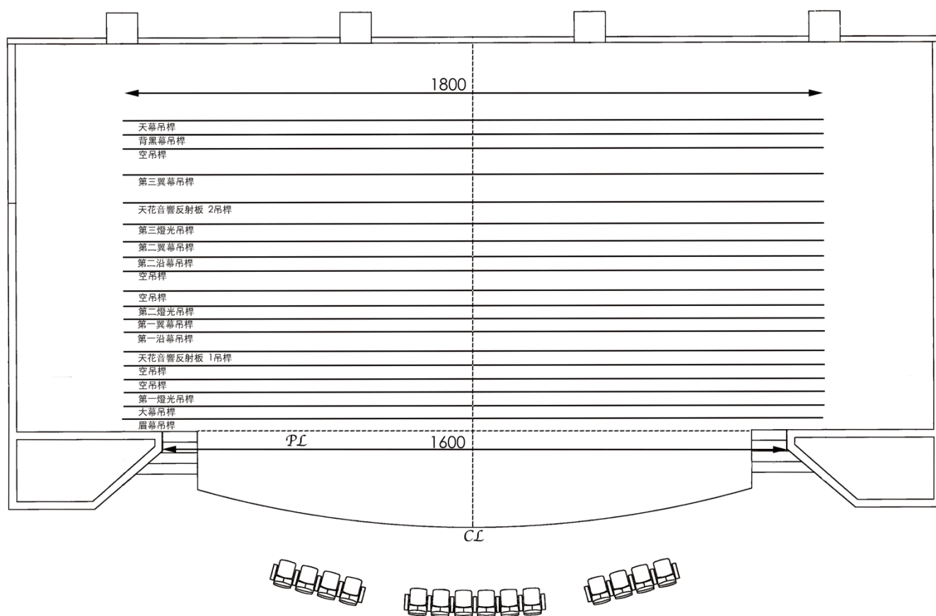
懸吊平面圖
