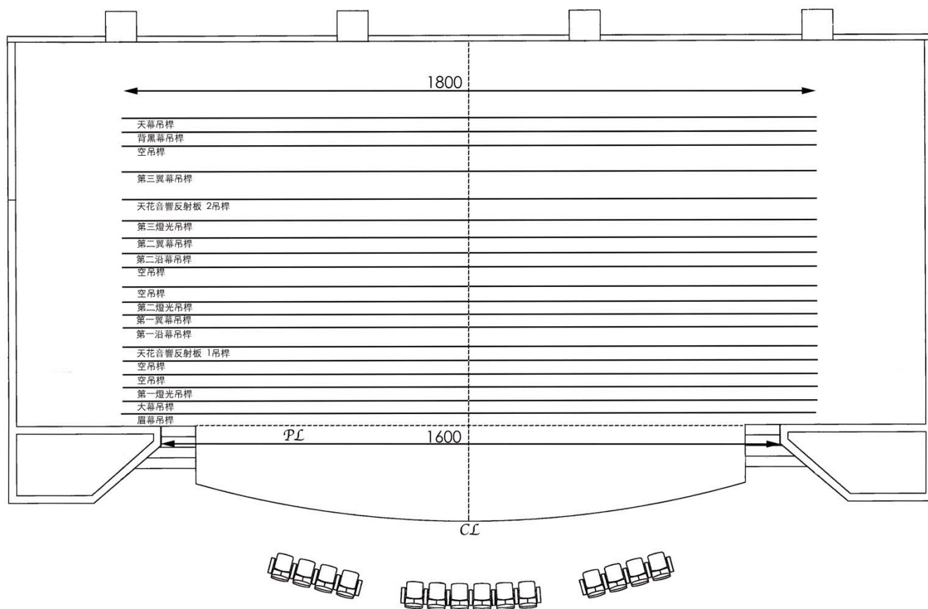
懸吊平面圖
