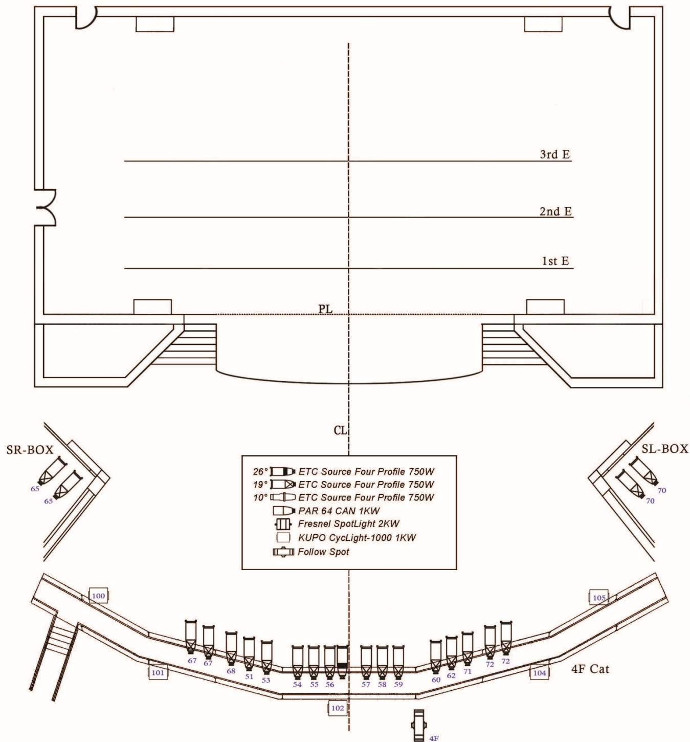
燈具配置圖
